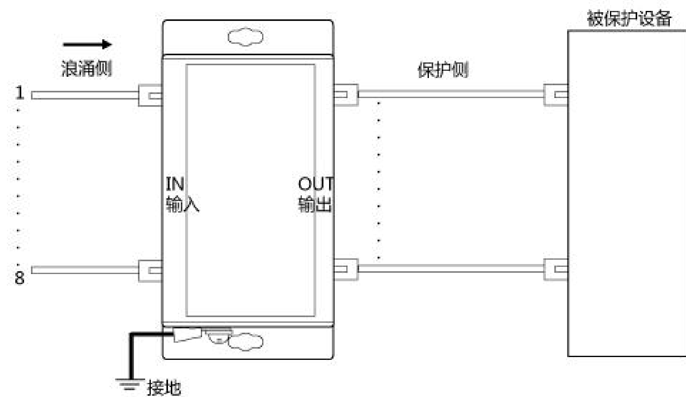
UT-N204G 接线示意图
