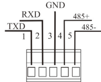
RS-232/RS-485输入 接口
