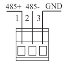
RS-485输出 接口
