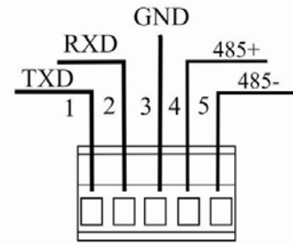
RS-232/RS-485输入 接口
