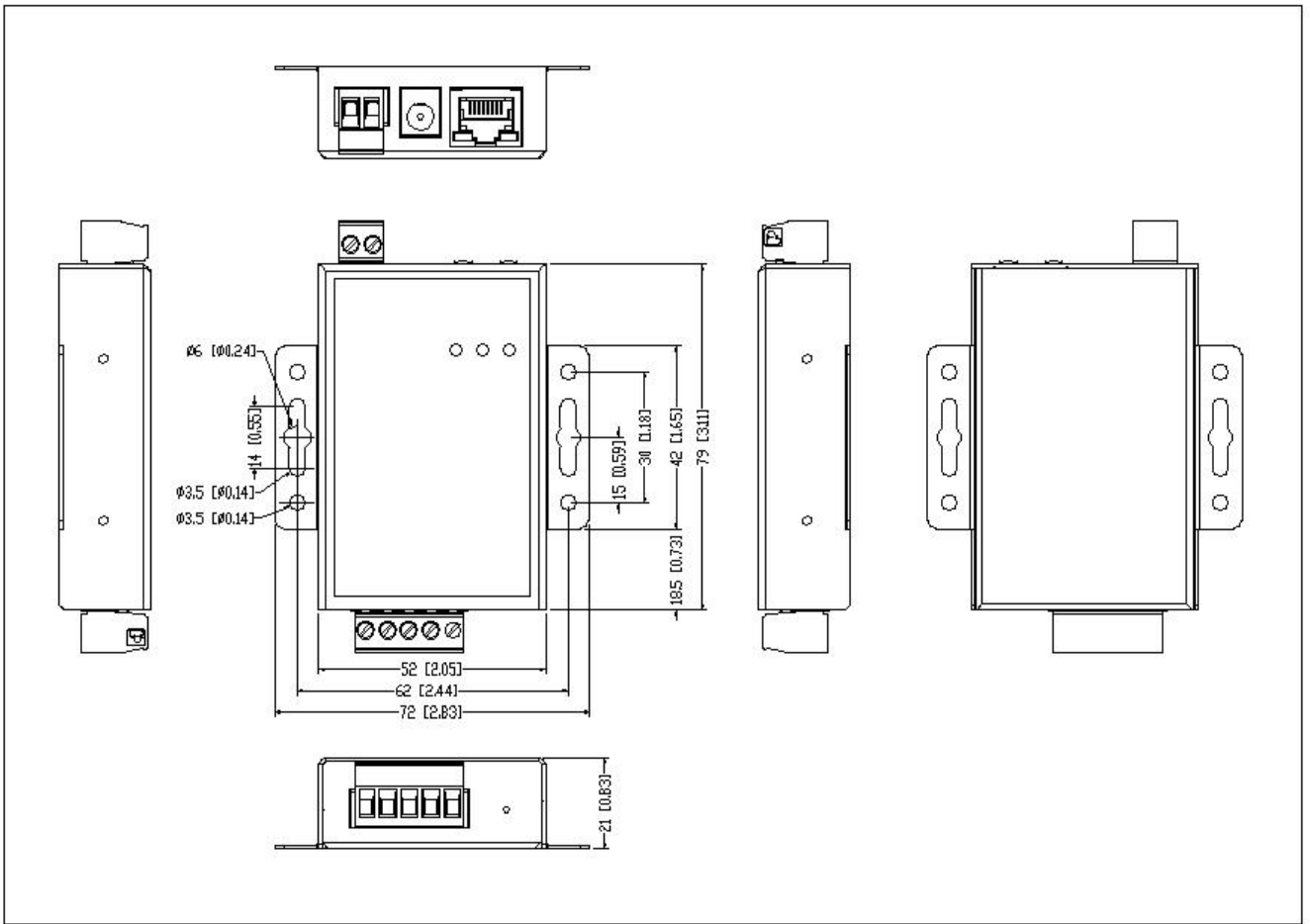
UT-6311M 外形尺寸图
