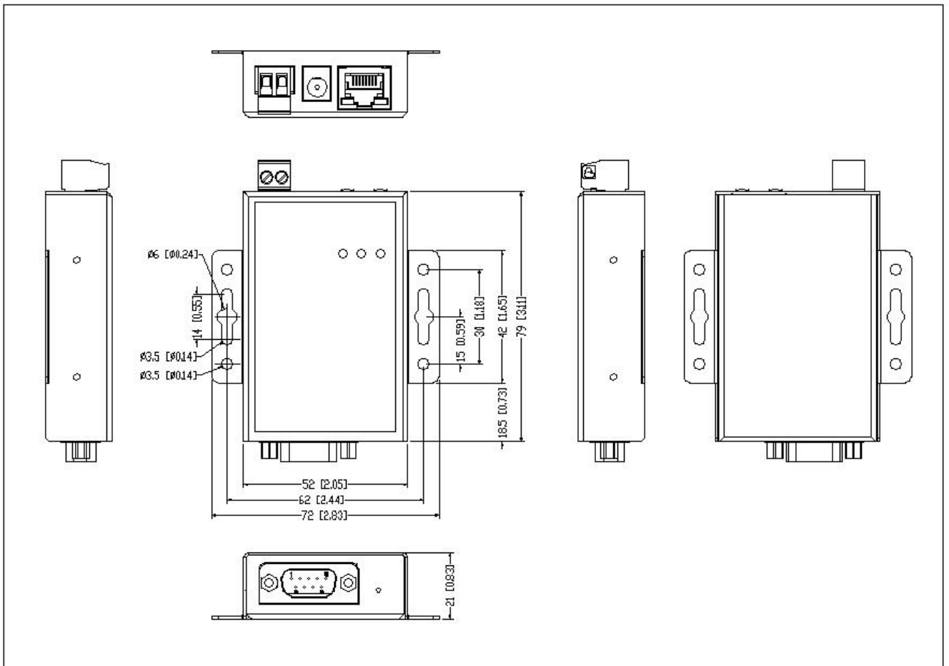
UT-6311C 外形尺寸图
