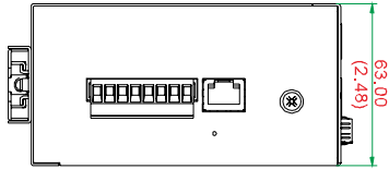
顶视图
