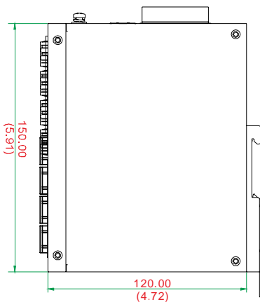
前视图
